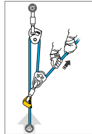
ホーリングシステム
