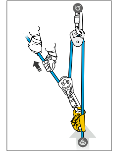
アッセンダー『ベーシック』を使用した引き上げシステム
